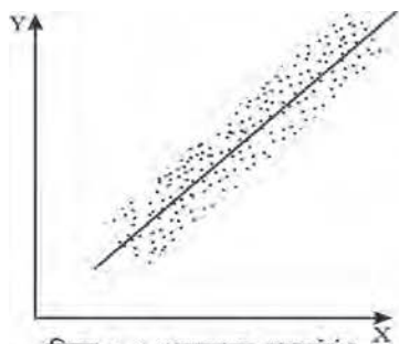
चित्र 6.1 धनात्मक सहसंबंध
