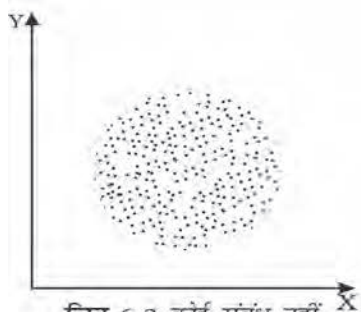
चित्र 6.3 कोई संबंध नहीं
