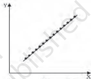
चित्र 6.4 पूर्ण धनात्मक सहसंबंध
