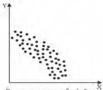
चित्र 6.7 ऋणात्मक गैर-रेखीय संबंध
