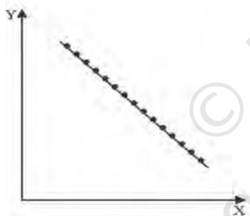
चित्र 6.5 पूर्ण ऋणात्मक सहसंबंध
